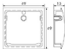
Model: SYJ3116 Material: Zinc Brush Nickel
