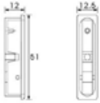
Model: SYJ3104 Material: Zinc Pearl Nickel
