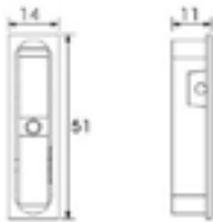
Model: SYJ3108 Material: Zinc Pearl Nickel
