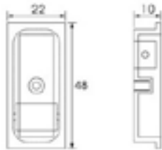
Model: SYJ3106 Material: Zinc Pearl Nickel
